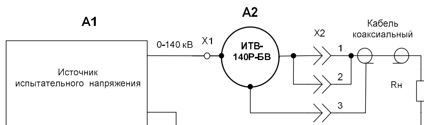
Рисунок 3. Схема подключения высокопотенциального блока ИТВ-140Р-БВ
