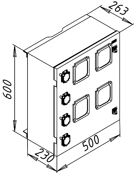
Шафа ARED-65-M4
