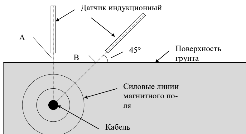
Рисунок 17. Определение глубины залегания кабеля.
