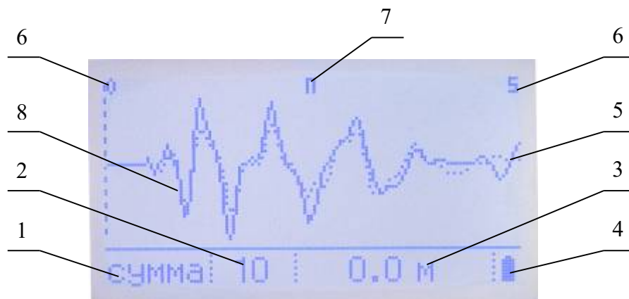
Рисунок 12. Меню режима автоматического накопления сигнала
